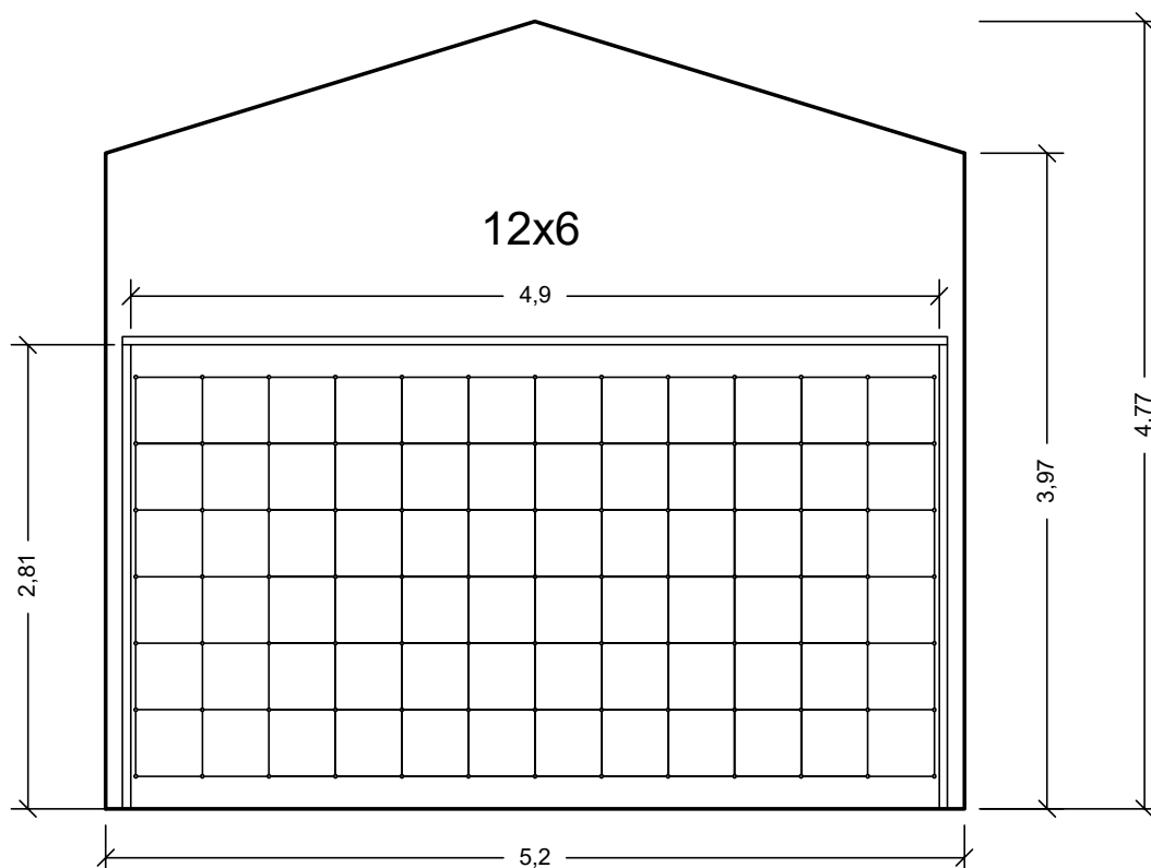
PROSPETTO STATO DI PROGETTO
